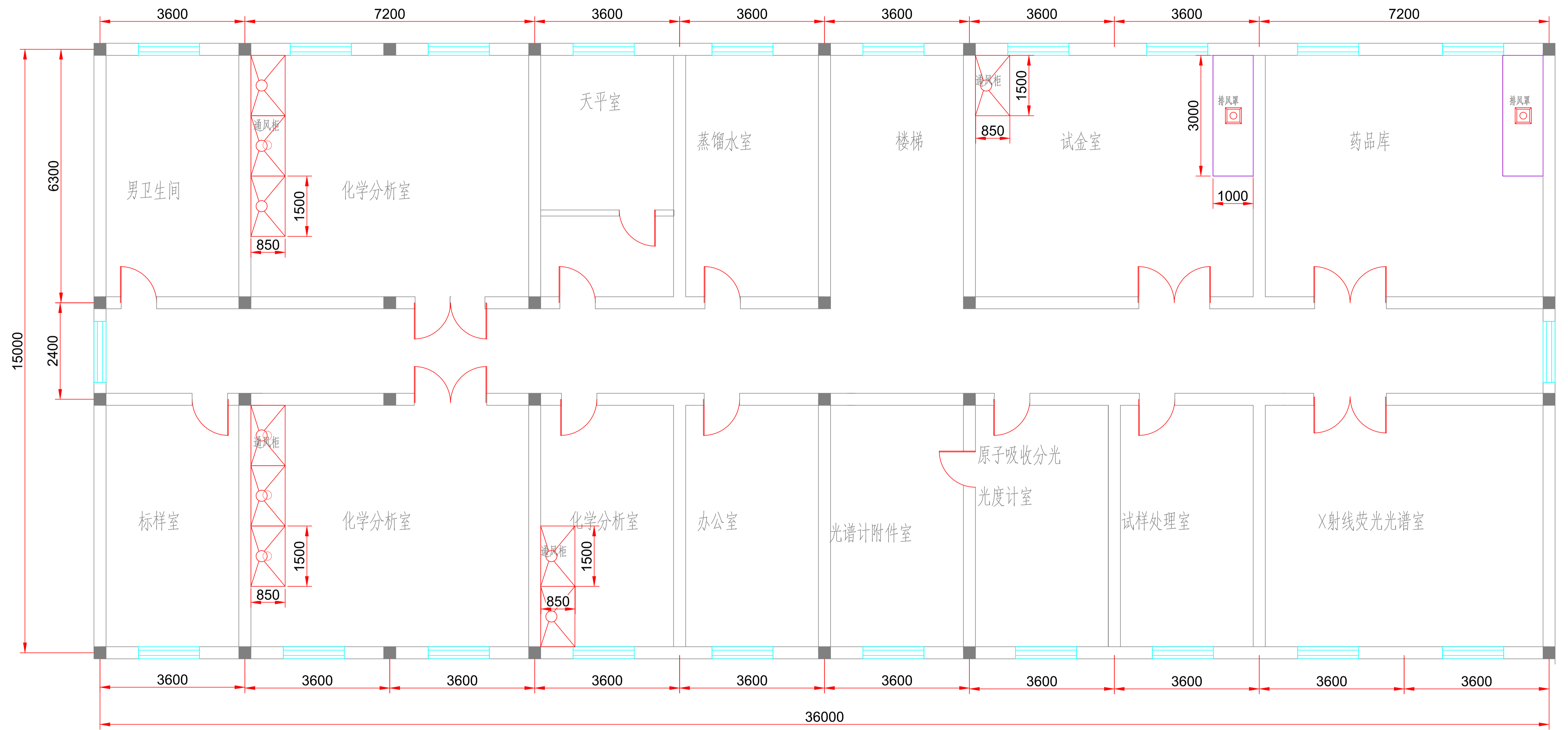
二层平面
